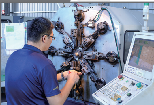
CNC multi-function forming machine CNC 多軸成型機
